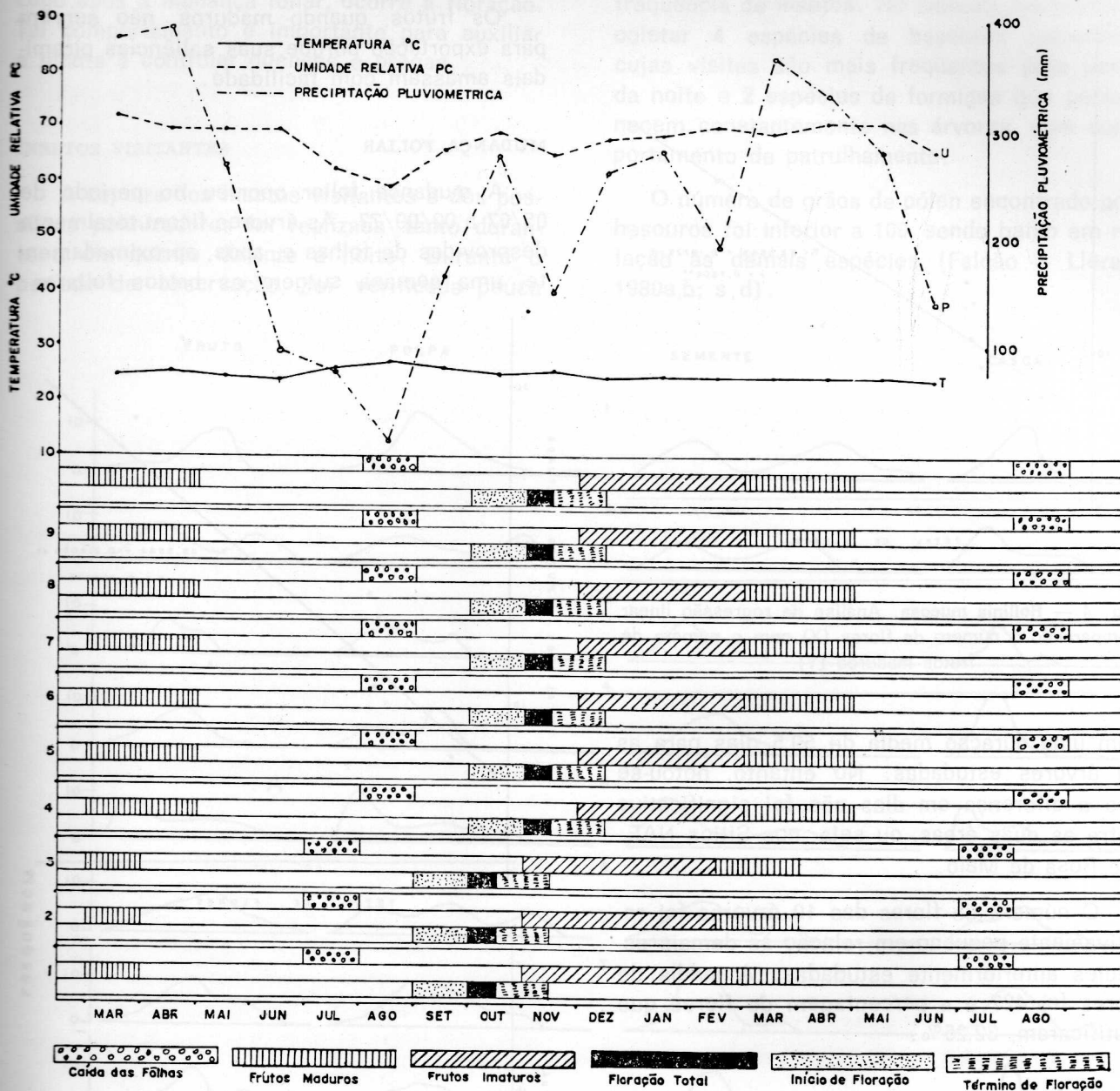
Fig. 3 — Rollinia mucosa . Quadro geral de floração, frutificação, produção e queda de folhas. Na parte superior, dados climatológicos para a área de Manaus (cf. Ribeiro, 1977); na parte inferior, dados fenológicos.
