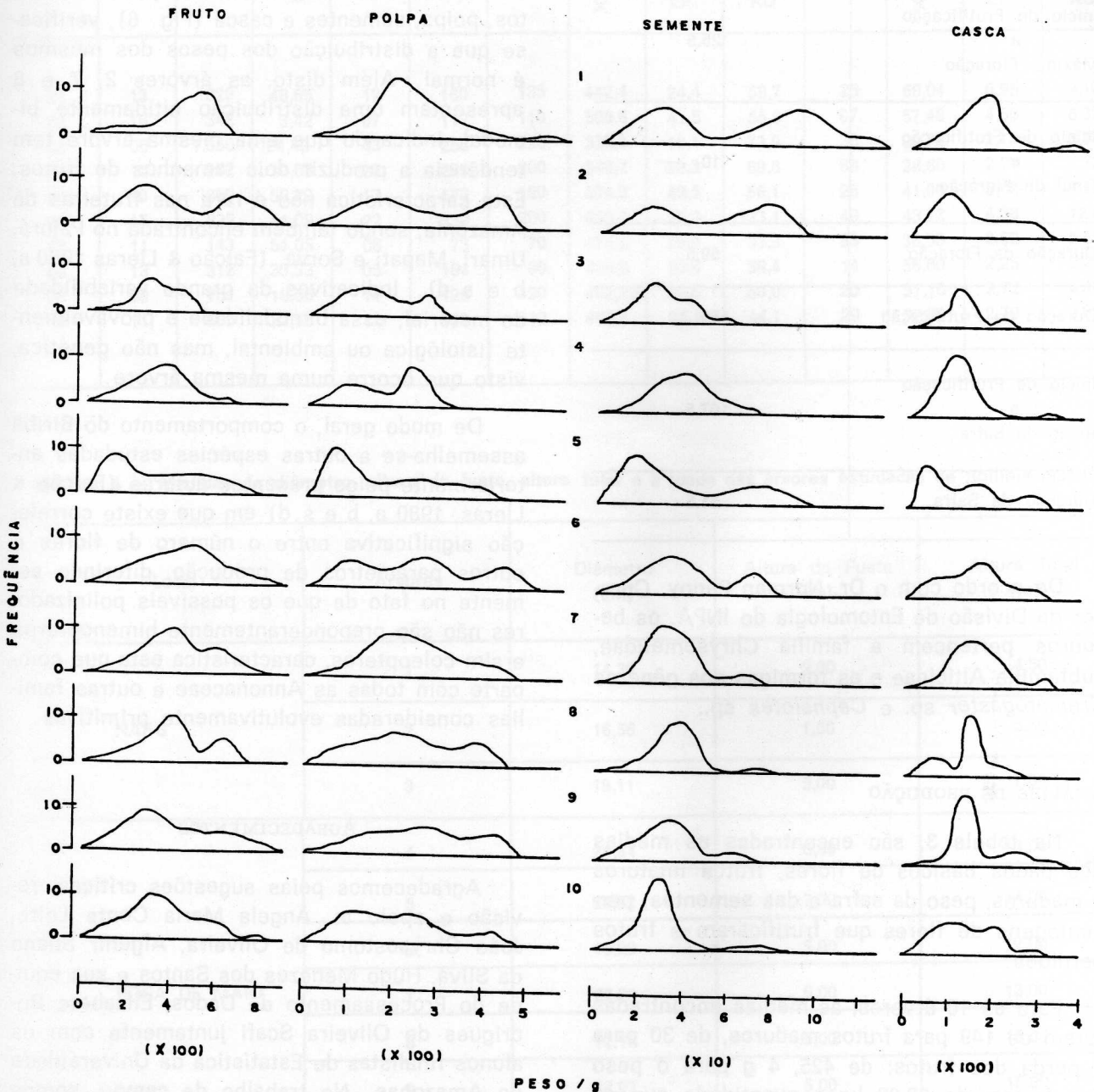
Fig. 6 — Rollinia mucosa . Freqüência de pesos de fruto total, polpa, sementes e casca das 10 árvores.
