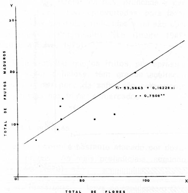
Fig. 4 — Rollinia mucosa . Análise de regressão linear comparando o número de flores (X) com o número de frutos maduros (Y).
