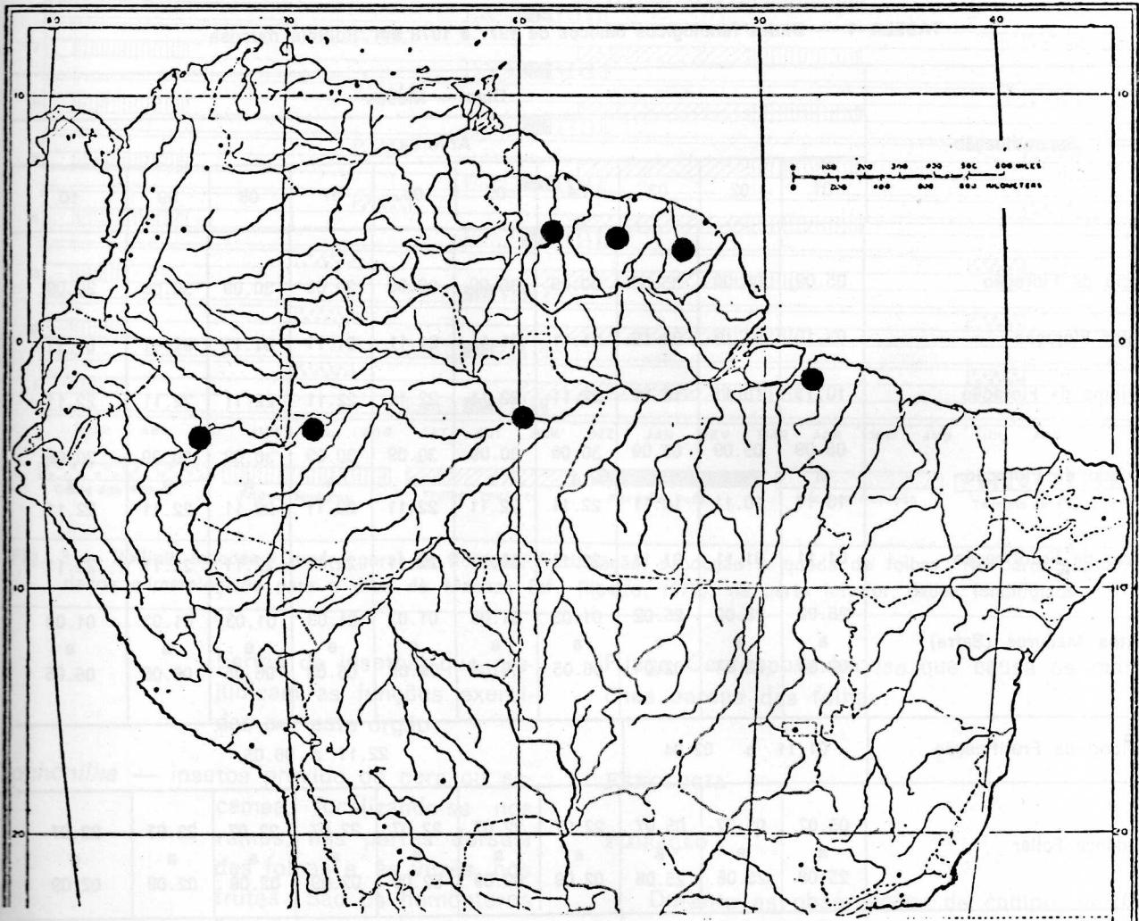
Fig. 2 — Distribuição geográfica conhecida de Rollinia mucosa , para a Amazônia.
