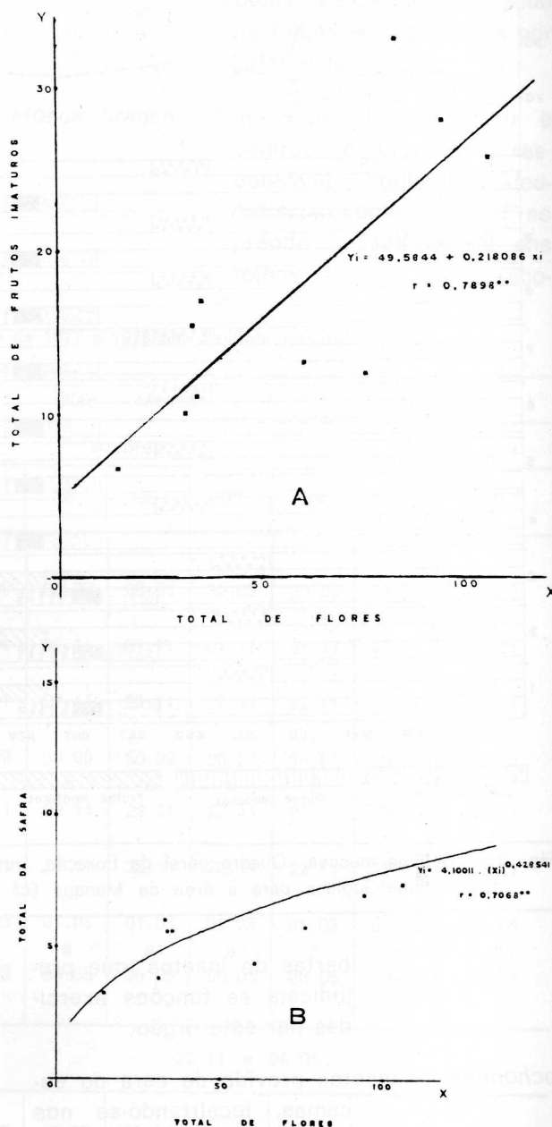
Fig. 5 — Rollinia mucosa . Análise de regressão linear: A, comparando o número de flores com o número de frutos imaturos; B, número de flores com peso significativo a nível de 1%, r = coeficiente de correlação entre X e Y.
