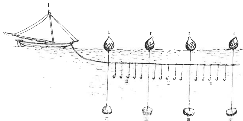
Fig. 3 — Esboço de um espinhel com seus componentes: I — bóias; II — anzóis; III — poitas. (Des. G. Leite)
